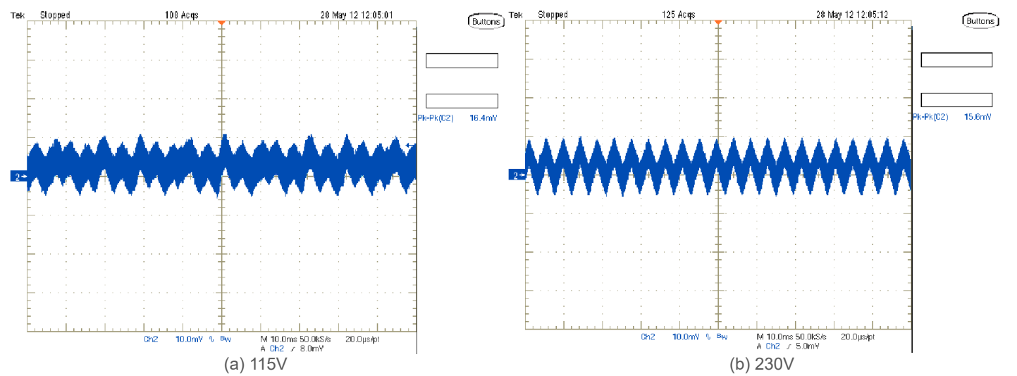
図 2 リップル&ノイズ例、20MHz BW
