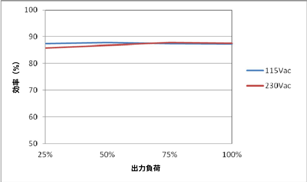
図 1 効率と出力負荷の比較
